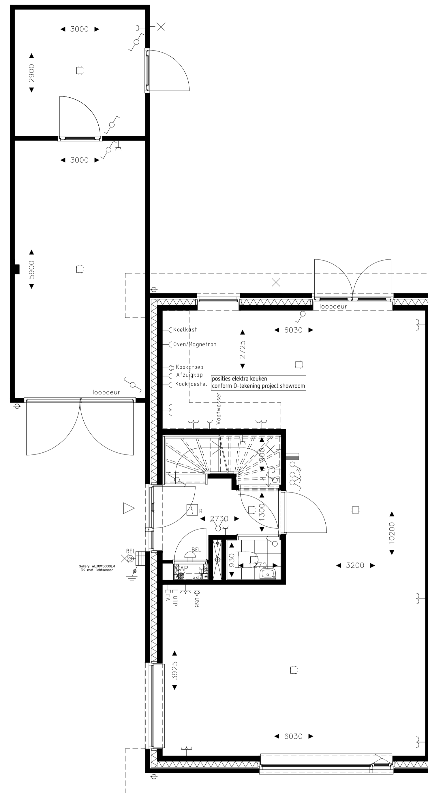
optie uitbouw berging met tuinberging plattegrond begane grond schaal 1:50
